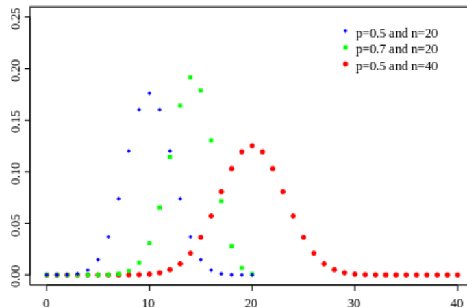
Binomial distribution
